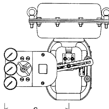
图 15 安装 HTP 定位器
