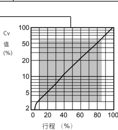
图 5. Cv 值 0.4 ~ 14 (等百分比特性)
