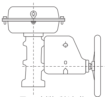
图 12 侧装手轮机构
