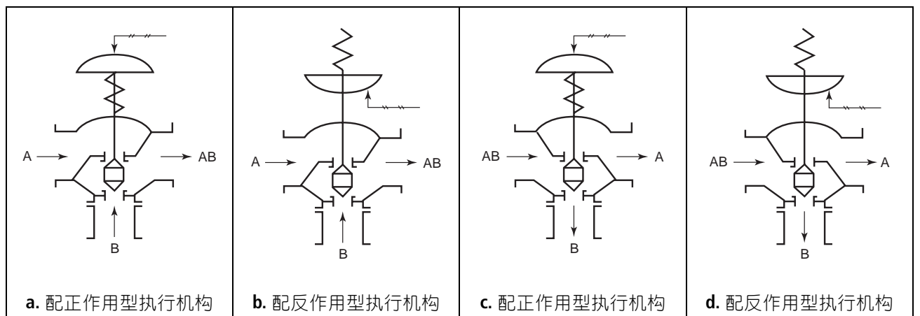
图 3 阀作用
