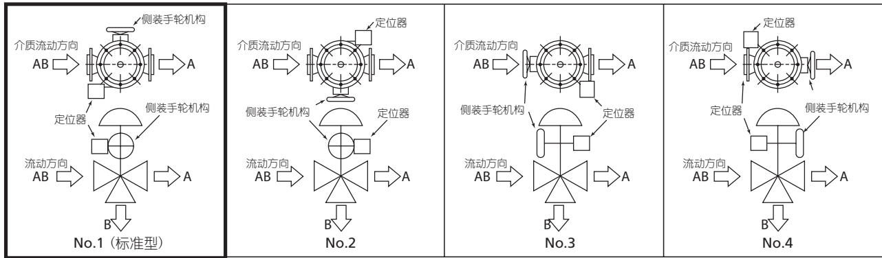
图 5 配管安装示意图
